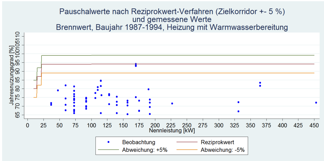
Abbildung 6: Vergleich nach Reziprokwert-Verfahren bestimmte-Pauschalwerte und Messwerte für Brennwert-Heizungsanlagen der Baujahre 1987-1994 mit Warmwasserbereitung. 4,2 % der Beobachtungen liegen im +/-5% Zielkorridor
