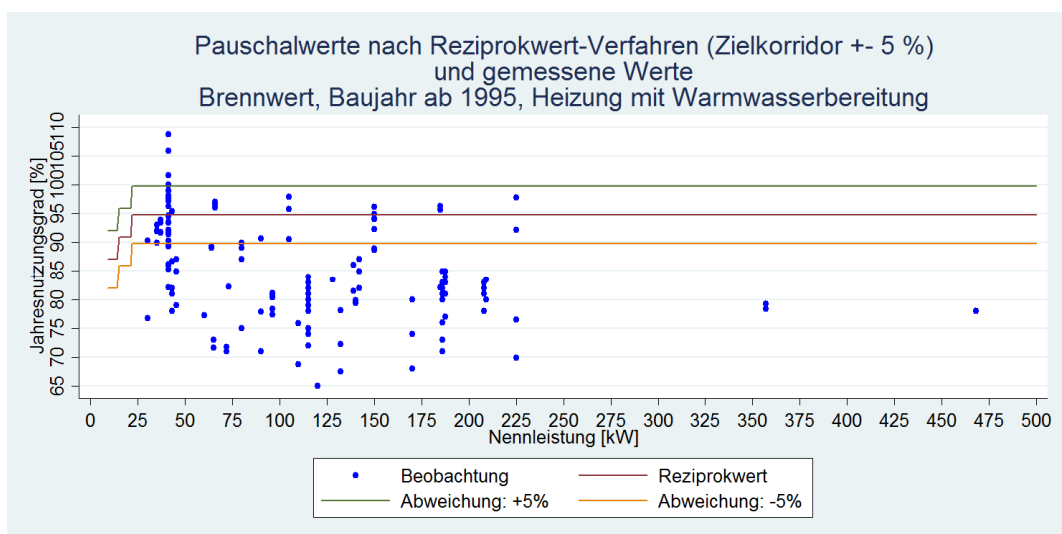
Abbildung 7: Vergleich nach Reziprokwert-Verfahren bestimmte-Pauschalwerte und Messwerte für Brennwert-Heizungsanlagen ab Baujahr 1995 mit Warmwasserbereitung. 28,9 % der Beobachtungen liegen im +/-5 % Zielkorridor.
