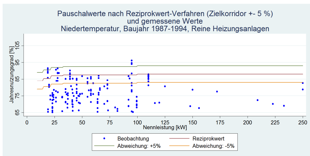
Abbildung 1: Vergleich nach Reziprokwert-Verfahren bestimmte-Pauschalwerte und Messwerte für NT-Heizungsanlagen BJ 1987-1994. 29,3 % der Beobachtungen liegen im \pm 5\% Intervall des Zielkorridors.
