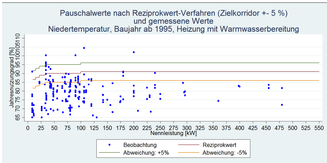
Abbildung 5: Vergleich nach Reziprokwert-Verfahren bestimmte-Pauschalwerte und Messwerte für NT-Heizungsanlagen Baujahr ab 1995 mit Warmwasserbereitung. 19,2 % der Beobachtungen liegen im +5% Intervall des Zielkorridors
