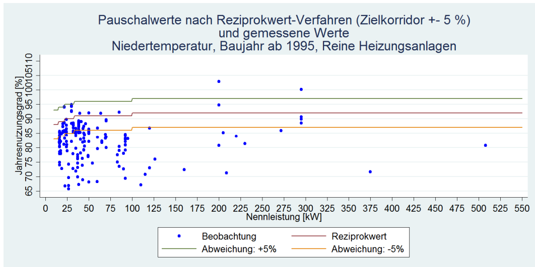
Abbildung 2: Vergleich nach Reziprokwert-Verfahren bestimmte-Pauschalwerte und Messwerte für NT-Heizungsanlagen BJ ab 1995. 32,6 % der Beobachtungen liegen im +5% Intervall des Zielkorridors.
