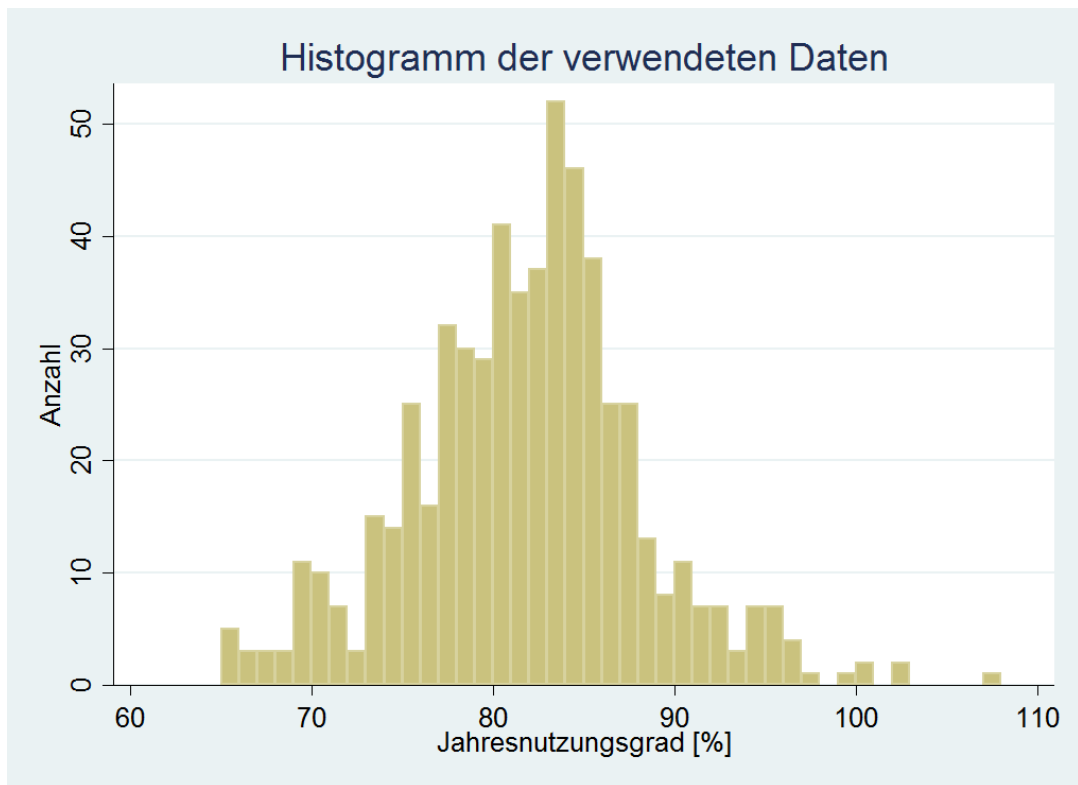
Abbildung 9: Histogramm des JNG der betrachteten Anlagen
