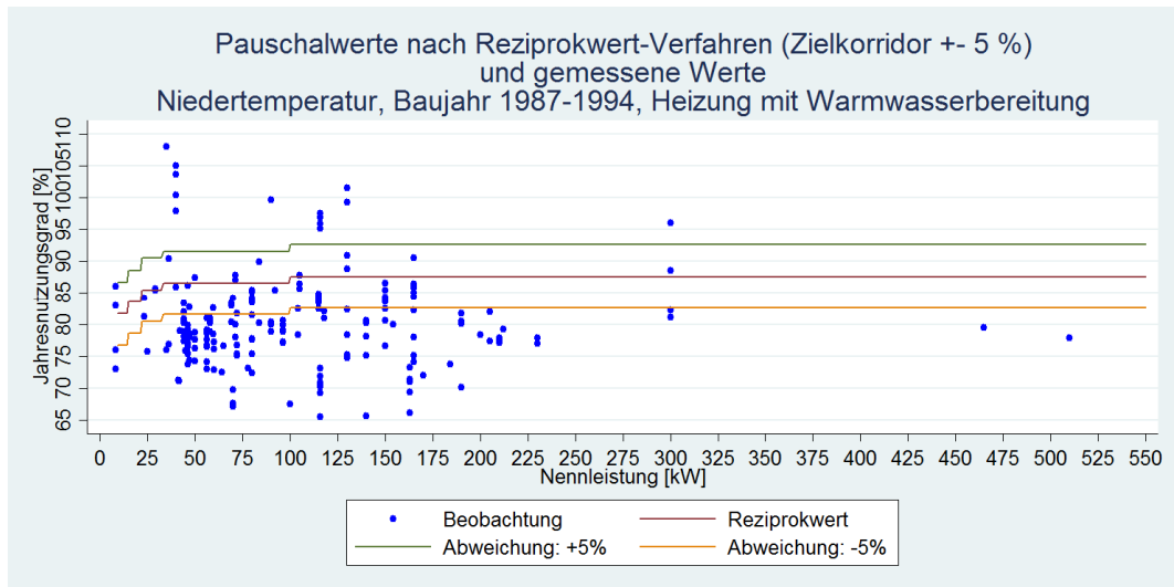
Abbildung 4: Vergleich nach Reziprokwert-Verfahren bestimmte-Pauschalwerte und Messwerte für NT-Heizungsanlagen Baujahr 1987-1994 mit Warmwasserbereitung. 24,8 % der Beobachtungen liegen im +5% Intervall des Zielkorridors
