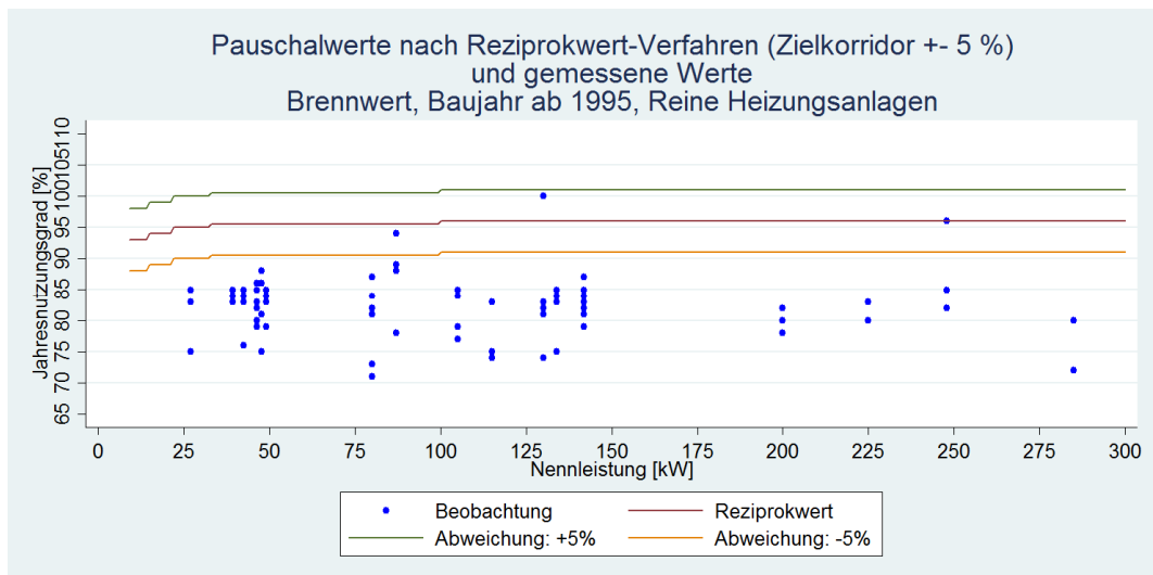
Abbildung 3: Vergleich nach Reziprokwert-Verfahren bestimmte-Pauschalwerte und Messwerte für reine Brennwert-Heizungsanlagen BJ ab 1995. 3,2 % der Beobachtungen liegen im +5% Intervall des Zielkorridors.
